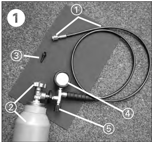
HW 100 mit Quick-Fill-Kartusche
